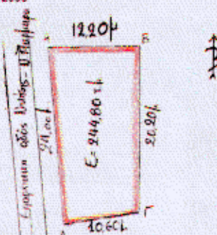
ΤΟΠΟΓΡΑΦΙΚΟ ΔΙΑΓΡΑΜΜΑ Δημόσιας Δασικής έκτασης εμβαδού 244,80 τ.μ. στη θέση «Κυραμαριά» περιοχής Δημ. Δ/τος Ν. Μαρμαρά Δήμου Σιθωνίας η οποία καταστράφηκε από πυρκαγιά που έγινε στις 24-6-2000
