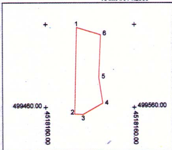
ΤΟΠΟΓΡΑΦΙΚΟ ΔΙΑΓΡΑΜΜΑ ΚΛΙΜΑΚΑ 1:2000
