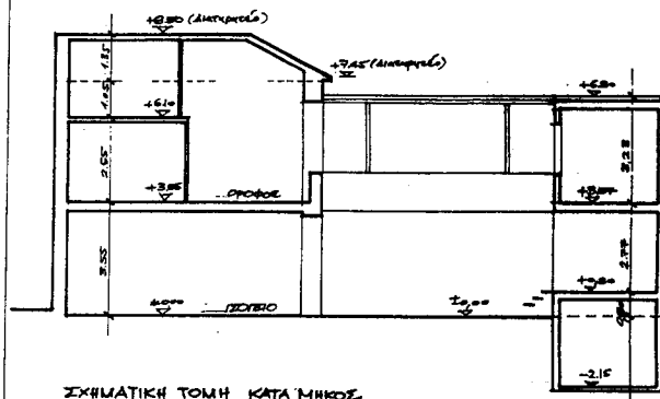
ΣΧΗΜΑΤΙΚΗ ΤΟΜΗ ΚΑΤΑ ΜΗΚΟΣ
