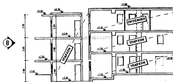
ΤΟΜΗ Α-Α 1/100
