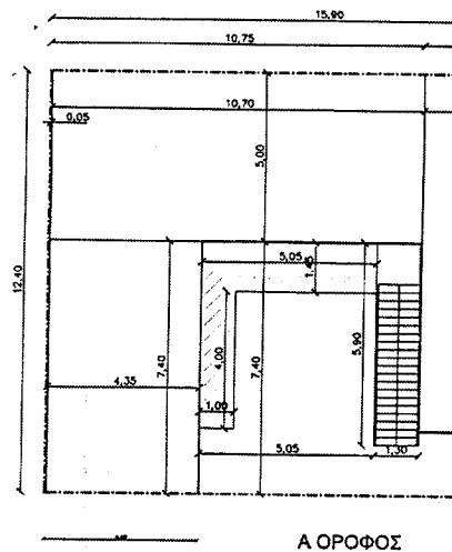
Α-ΟΡΟΦΟΣ
