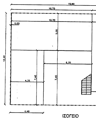
ΙΣΟΓΕΙΟ
