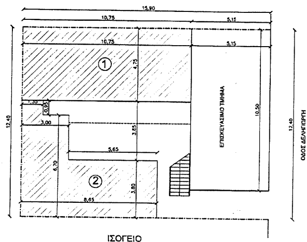
ΙΣΟΓΕΙΟ
