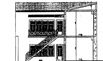
ΤΟΜΗ Α-Α'
