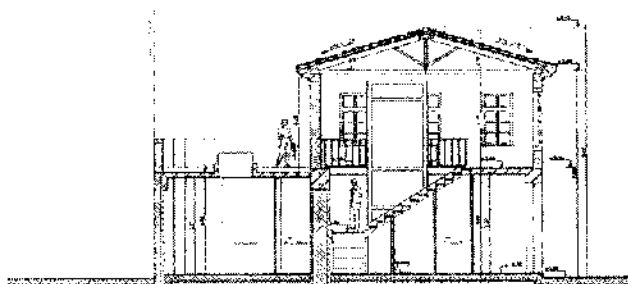
ΤΟΜΗ Γ-Γ
