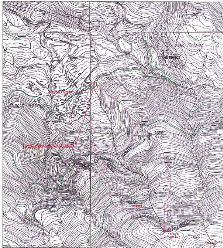
ΤΟΠΟΓΡΑΦΙΚΟ ΔΙΑΓΡΑΜΜΑ ΠΕΡΙΟΧΗΣ 1:5000
