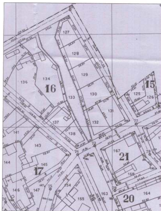
ΤΟΠΟΓΡΑΦΙΚΟ ΕΥΡΥΤΕΡΗΣ ΠΕΡΙΟΧΗΣ ΚΛΙΜΑΚΑ 1:2000
