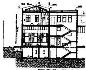
ΣΥΝΑΝΤΗΣΗ ΤΟΜΗ ΚΤΙΡΙΟΥ (B-B)
