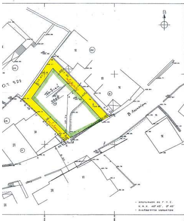
Σ. ΡΥΘΜΟΤΟΜΙΚΟΥ 1990 ΚΑΛΑ 1 : 2000
