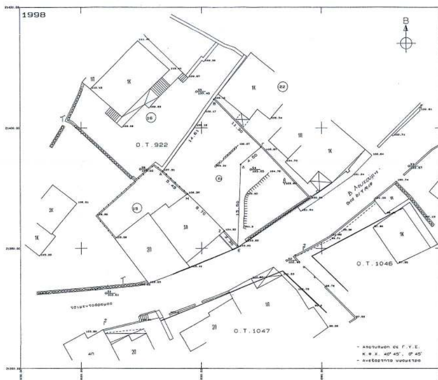
ΑΠΟΦΑΣΗ 1998 ΚΑΙΜΑΚΑ 1 : 1000
