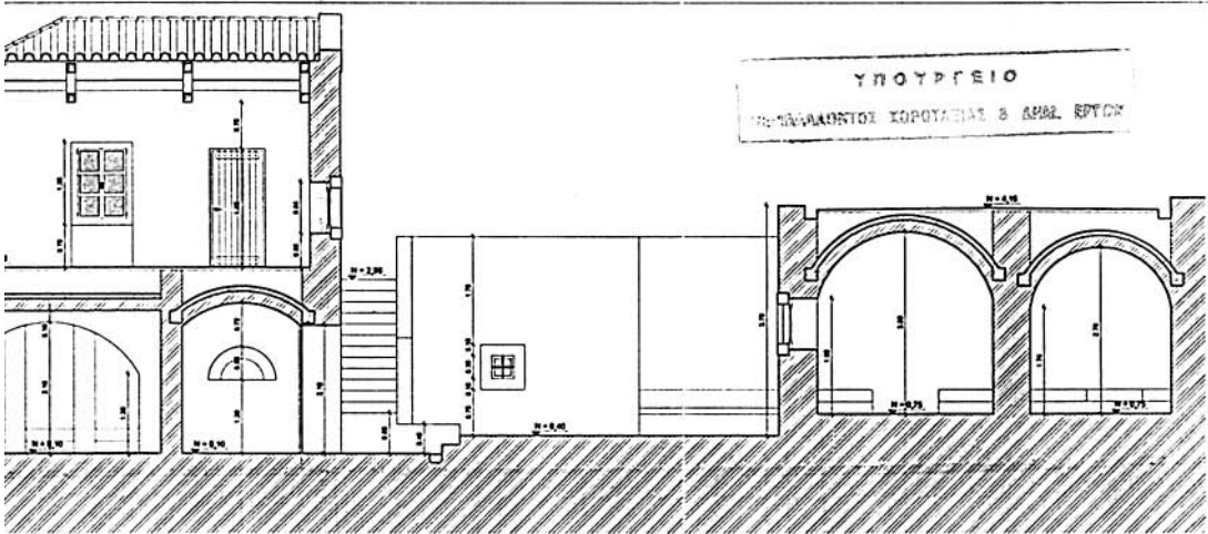
ΤΟΜΗ Α-Α
