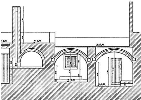
ΤΟΜΗ Β-Β
