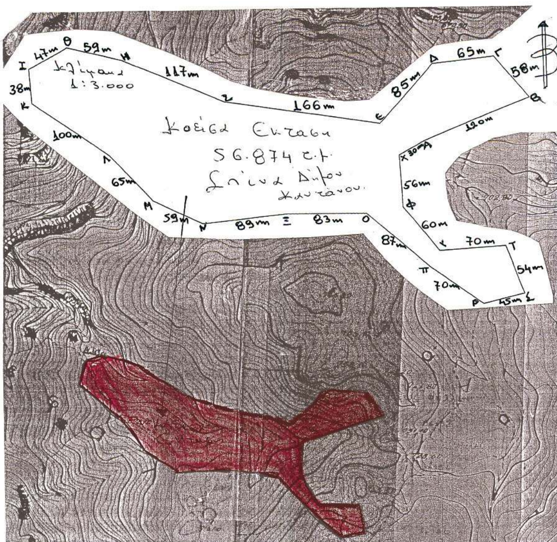
ΤΟΠΟΓΡΑΦΙΚΟ ΔΙΑΓΡΑΜΜΑ
