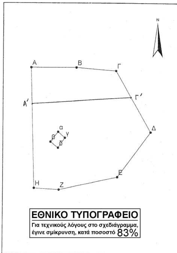
ΤΟΠΟΓΡΑΦΙΚΟ ΔΙΑΓΡΑΜΜΑ
