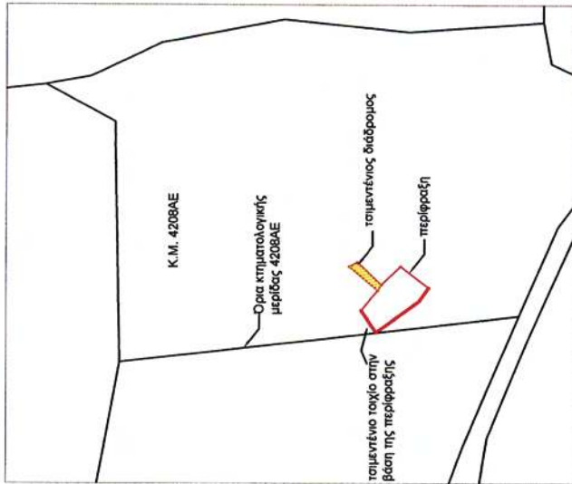
ΑΠΟΣΠΑΣΜΑ ΤΟΠΟΓΡΑΦΙΚΟΥ ΔΙΑΓΡΑΜΜΑΤΟΣ ΤΗΣ Κ.Μ. 4208ΑΕ ΓΑΙΩΝ ΑΡΧΑΓΓΕΛΟΥ
