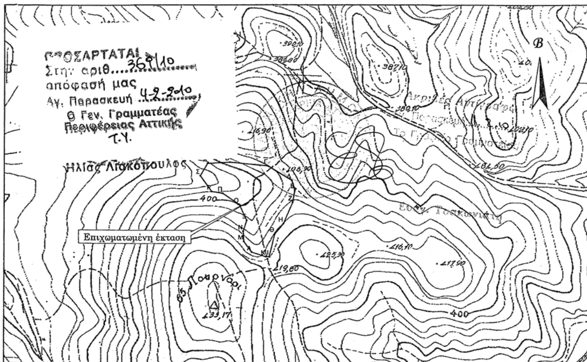
ΤΟΠΟΓΡΑΦΙΚΟ ΔΙΑΓΡΑΜΜΑ
