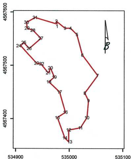
ΤΟΠΟΓΡΑΦΙΚΟ ΔΙΑΓΡΑΜΜΑ Κλίμακα 1:3.000
