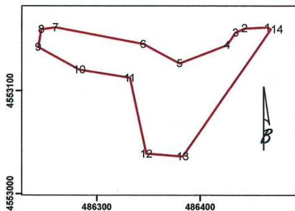
ΤΟΠΟΓΡΑΦΙΚΟ ΔΙΑΓΡΑΜΜΑ Κλίμακα 1:3.000
