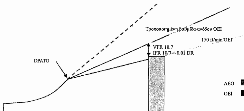
Σχήμα 6 – Επιδόσεις Τάξης 2 (επαυξημένη βαθμίδα ανόδου)
