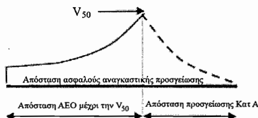
Σχήμα 10 – Απόσταση ασφαλούς αναγκαστικής προσγείωσης Κατηγορίας Β ( V_{50} )
