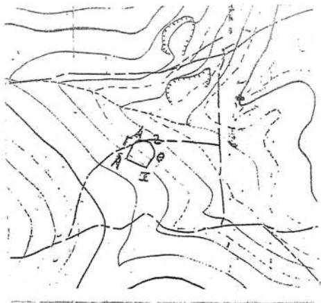
Η έκταση υπό στοιχεία (Α, Β, Γ, Δ, Ε, Ζ, Η, Θ, Ι, Α) κλίμ 1:500
