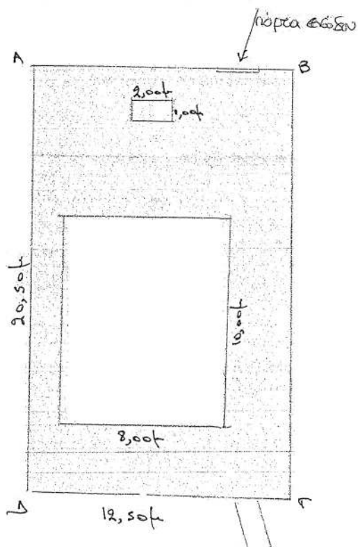
Τοπογραφικό διάγραμμα Κλ. 1:200
