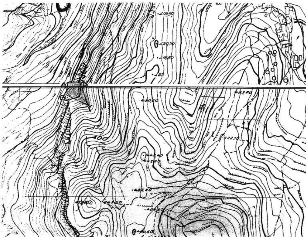
ΤΟΠΟΓΡΑΦΙΚΟ ΔΙΑΓΡΑΜΜΑ
