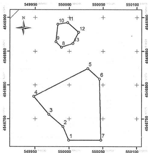
ΤΟΠΟΓΡΑΦΙΚΟ ΔΙΑΓΡΑΜΜΑ ΚΛΙΜΑΚΑΣ 1:2.000
