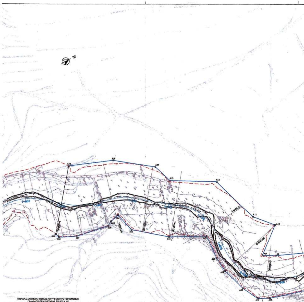
ΠΙΝΑΚΑΣ ΣΥΝΤΕΤΑΓΜΕΝΩΝ ΚΟΡΥΦΩΝ ΠΡΟΤΙΝΟΜΕΝΩΝ ΓΡΑΜΜΩΝ ΟΡΙΣΘΕΝΕΙΣ ΣΕ ΕΣΤ. 97
