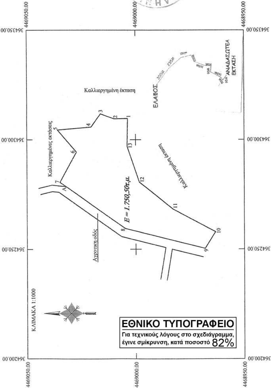
ΤΟΠΟΓΡΑΦΙΚΟ ΔΙΑΓΡΑΜΜΑ ΕΚΤΑΣΗΣ ΣΤΟΙΧΕΙΩΝ 1, 2, 3, ..., 12, 13, 1 ΚΑΙ ΕΜΒΑΔΟΥ Ε= 1.750,50τ.μ. ΣΤΗ ΔΑΣΙΚΗ ΘΕΣΗ "ΠΗΓΑΛΙΑ" ΤΗΣ ΤΟΠΙΚΗΣ ΚΟΙΝΟΤΗΤΑΣ ΕΛΛΑΦΟΥ ΤΟΥ ΔΗΜΟΥ ΚΑΤΕΡΙΝΗΣ Ν. ΠΙΕΡΙΑΣ
