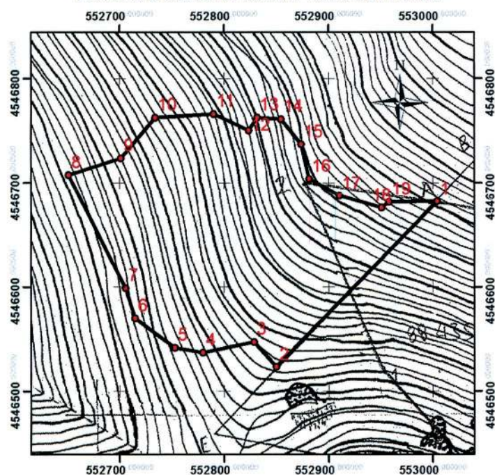
ΤΟΠΟΓΡΑΦΙΚΟ ΔΙΑΓΡΑΜΜΑ - ΚΛΙΜΑΚΑ 1:4.000
