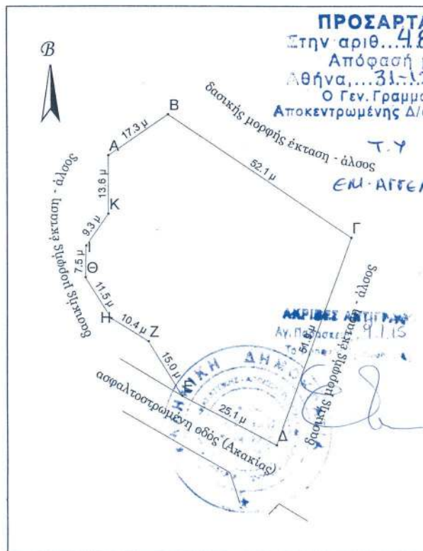
ΤΟΠΟΓΡΑΦΙΚΟ ΔΙΑΓΡΑΜΜΑ
