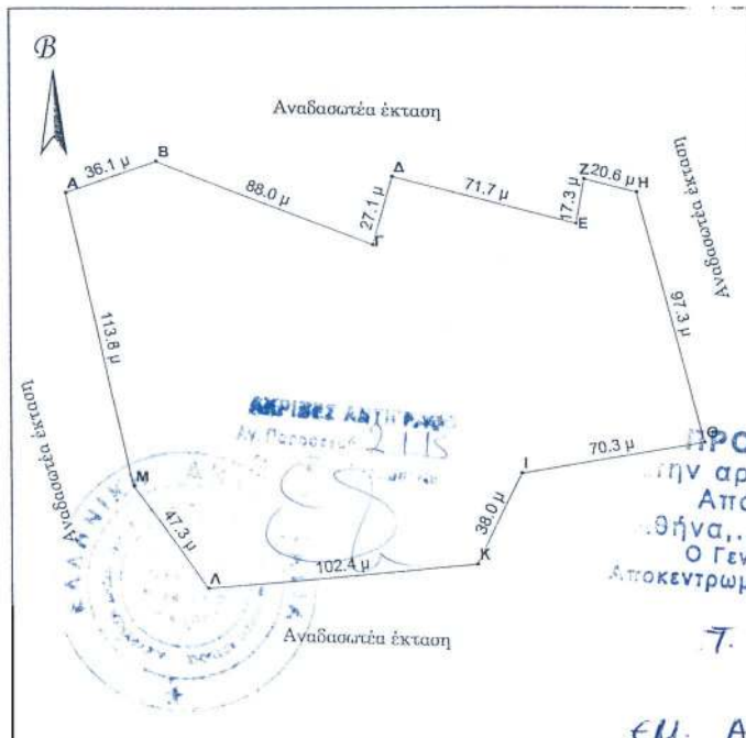
ΤΟΠΟΓΡΑΦΙΚΟ ΔΙΑΓΡΑΜΜΑ
