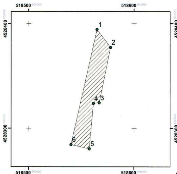
ΤΟΠΟΓΡΑΦΙΚΟ ΔΙΑΓΡΑΜΜΑ - ΚΛΙΜΑΚΑ 1:1.500
