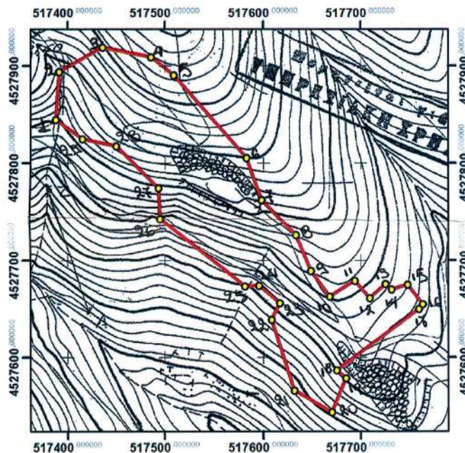
ΤΟΠΟΓΡΑΦΙΚΟ ΔΙΑΓΡΑΜΜΑ Α - ΚΛΙΜΑΚΑ 1:2.000
