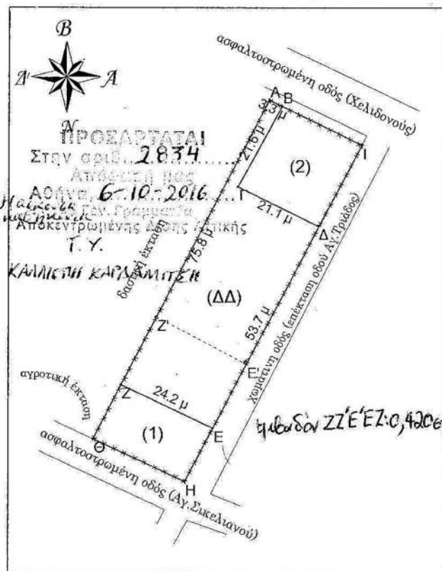
ΤΟΠΟΓΡΑΦΙΚΟ ΔΙΑΓΡΑΜΜΑ (κλίμ. 1:1000)
