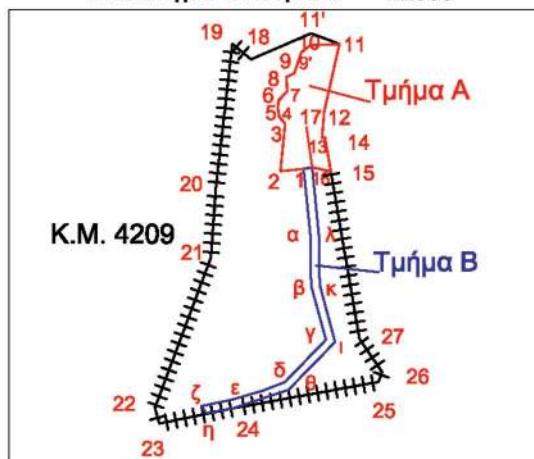
Ανάπτυγμα σε κλίμακα 1:2000
