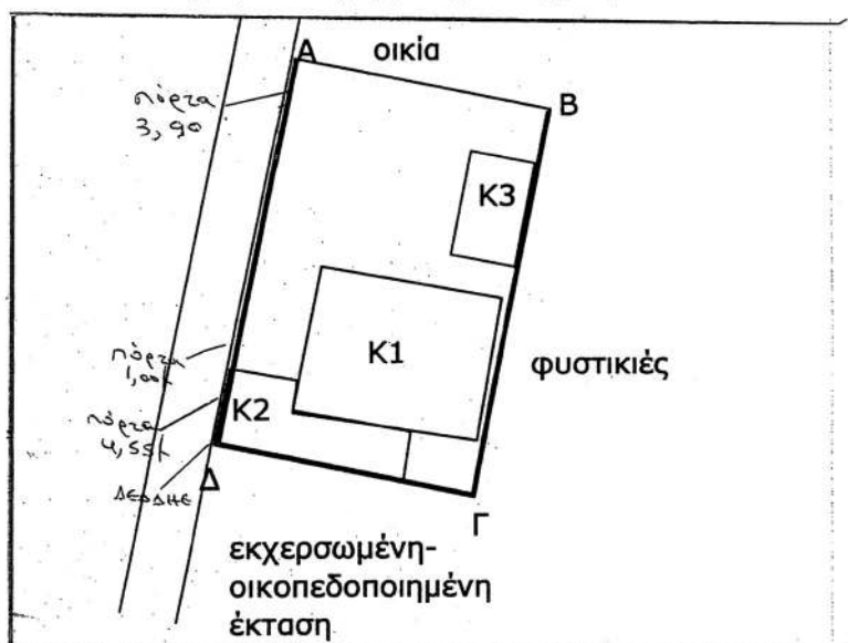
Τοπογραφικό Διάγραμμα της έκτασης κλιμ. 1:500
