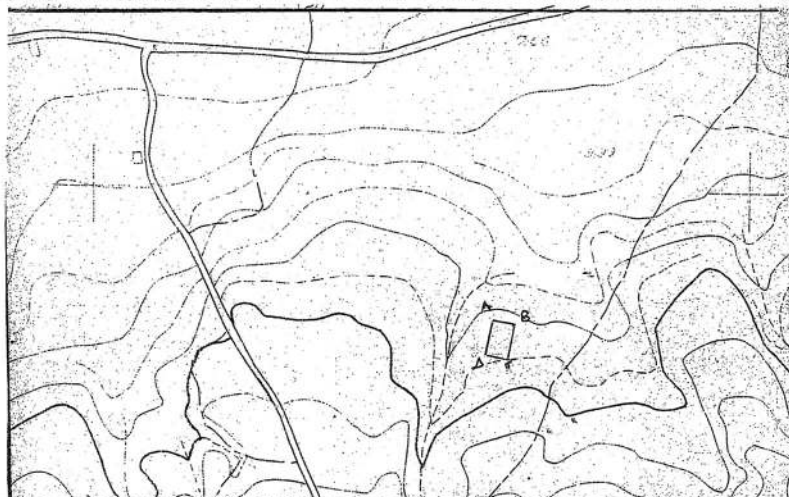
Τοπογραφικό Διάγραμμα της έκτασης κλιμ. 1:500
