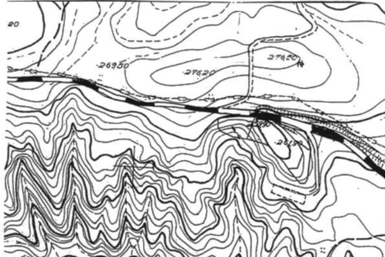
Τοπογραφικό Διάγραμμα της έκτασης κλίμ. 1:2000
