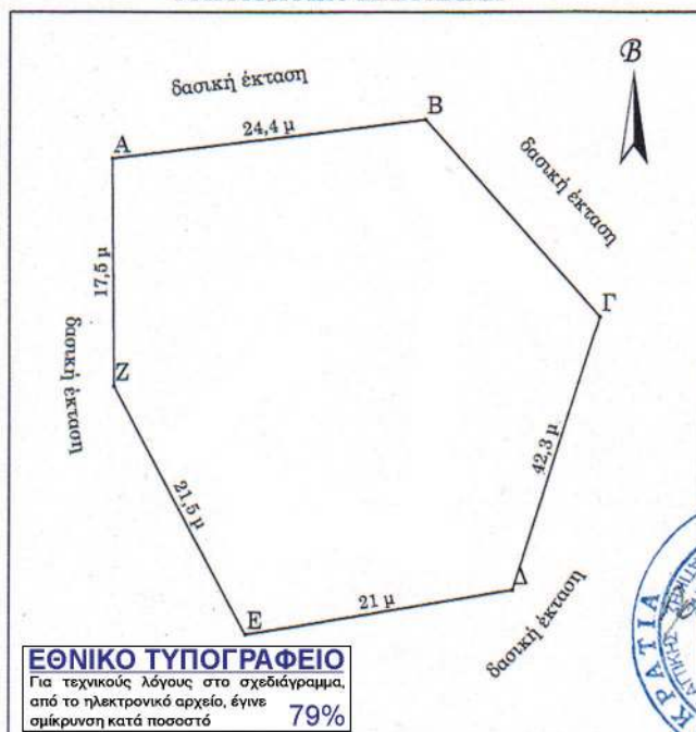
ΤΟΠΟΓΡΑΦΙΚΟ ΔΙΑΓΡΑΜΜΑ
