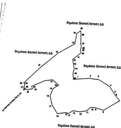
ΤΟΠΟΓΡΑΦΙΚΟ ΔΙΑΓΡΑΜΜΑ κλίμ.: 1:10.000
