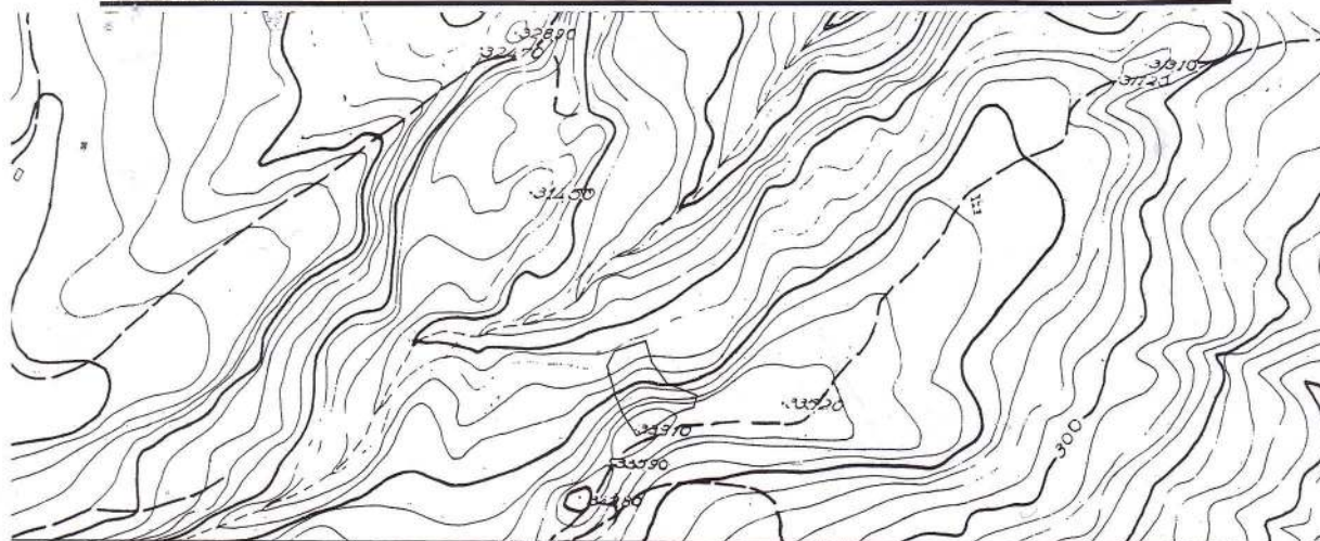
Τοπογραφικό Διάγραμμα της έκτασης κλιμ. 1:1000
