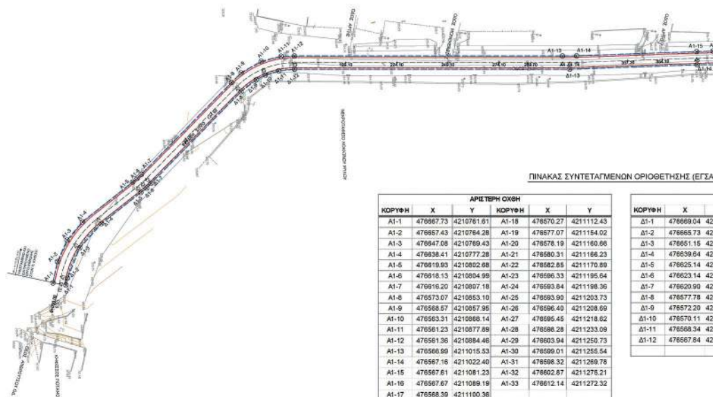
ΠΙΝΑΚΑΣ ΣΥΝΤΕΤΑΓΜΕΝΩΝ ΟΡΙΟΘΕΤΗΣΗΣ (ΕΓΓΙΑ 87)
