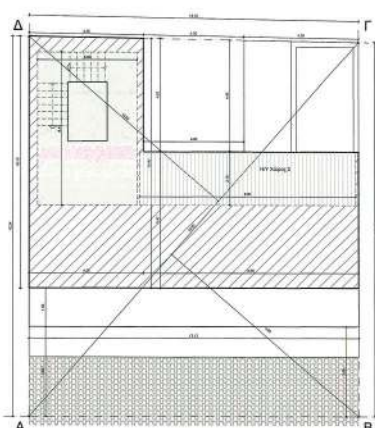
ΔΙΑΓΡΑΜΜΑ ΚΑΤΟΨΗΣ Δ' ΟΡΟΦΟΥ (προσθήκη)
