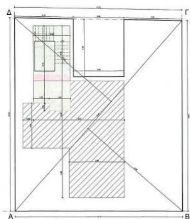
ΔΙΑΓΡΑΜΜΑ ΚΑΤΩΝΗΣ ΥΠΟΓΕΙΟΥ
