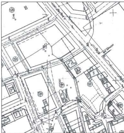
ΑΠΟΣΠΑΣΜΑ ΙΣΧΥΝΤΟΣ ΡΥΘΜΟΤΟΜΙΚΟΥ ΣΧΕΔΙΟΥ ΚΛΙΜΑΚΑ 1:1000
