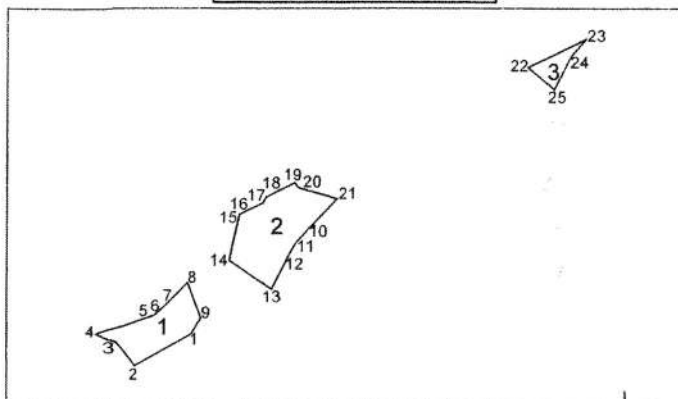
ΤΟΠΟΓΡΑΦΙΚΟ ΔΙΑΓΡΑΜΜΑ ΚΛΙΜΑΚΑ 1:2.500
