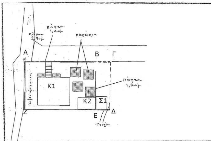
Τοπογραφικό Διάγραμμα της έκτασης κλίμ. 1:500
