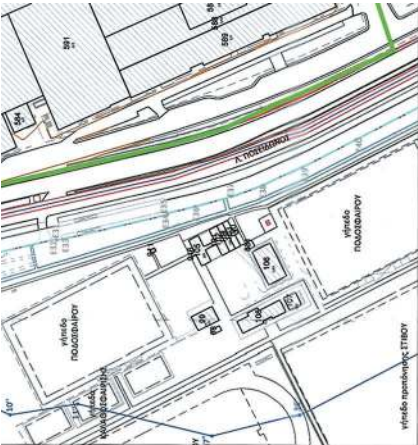
ΠΕΡΙΟΧΗ Δ_ΚΛΙΜΑΚΑ 1:200
