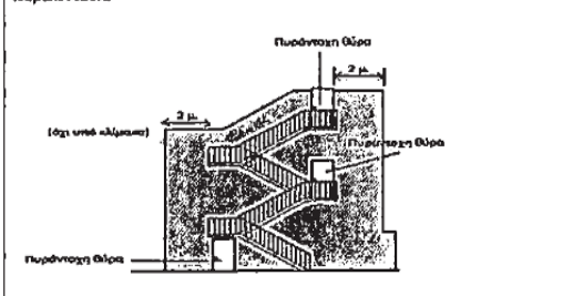
Σχήμα 23: Πυραντίσταση εξωτερικών τοίχων – θυρών και επέκταση αυτής για εξωτερικά κλιμακοστάσια
