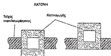
Σχήμα 21: Τυπική διάταξη πυράντοχων διαφραγμάτων (damper)
