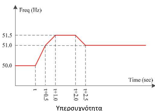
Εικ. 1: Καμπύλες ικανότητας αντοχής των μονάδων ηλεκτροπαραγωγής σε ρυθμούς μεταβολής συχνότητας συστήματος.
