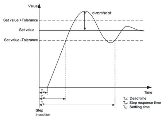
Εικ. 2 : ορισμοί παραμέτρων χρονικής απόκρισης μεταβλητής
