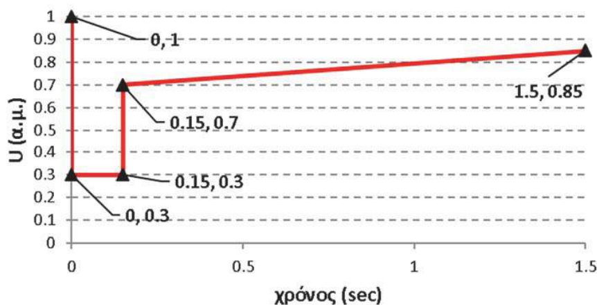
Εικ. 1: προφίλ ελάχιστης πολικής τάσεως στο σημείο σύνδεσης – χρόνου ικανότητας αδιάλειπτης λειτουργίας σε συμμετρικό σφάλμα για σύγχρονες γεννήτριες ηλεκτροπαραγωγής τύπου Β
