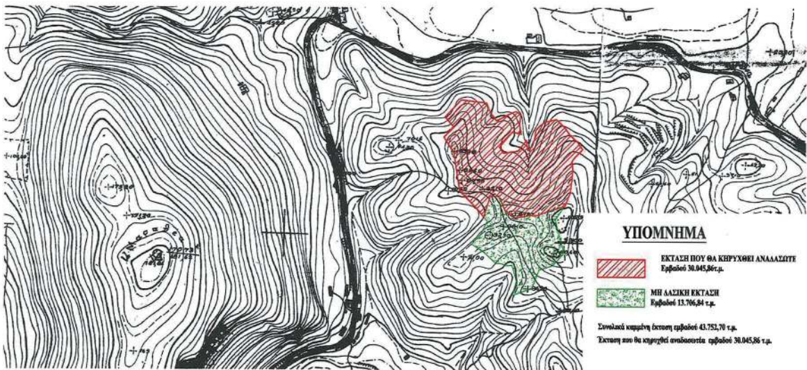
ΤΟΠΟΓΡΑΦΙΚΟ ΔΙΑΓΡΑΜΜΑ ΚΛΙΜΑΚΑΣ 1:2.500 ΤΗΣ ΕΚΤΑΣΗΣ ΠΟΥ ΚΑΗΚΕ ΣΤΙΣ 15-07-2019 ΚΑΙ ΘΑ ΚΗΡΥΧΘΕΙ ΑΝΑΛΑΣΩΤΕΑ ΣΤΗ ΘΕΣΗ ΠΑΣΣΑΒΑΣ ΤΗΣ ΤΟΠΙΚΗΣ ΚΟΙΝΟΤΗΤΑΣ ΧΩΣΙΑΡΙΟΥ ΤΟΥ ΔΗΜΟΥ ΑΝΑΤΟΛΙΚΗΣ ΜΑΝΗΣ.
