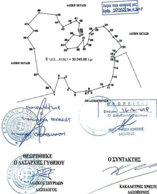
ΤΟΠΟΓΡΑΦΙΚΟ ΔΙΑΓΡΑΜΜΑ ΚΛΙΜΑΚΑΣ 1:2.500 ΤΗΣ ΕΚΤΑΣΗΣ ΠΟΥ ΚΑΗΚΕ ΣΤΙΣ 15-07-2019 ΚΑΙ ΘΑ ΚΗΡΥΧΘΕΙ ΑΝΑΛΑΣΩΤΕΑ ΣΤΗ ΘΕΣΗ ΠΑΣΣΑΒΑΣ ΤΗΣ ΤΟΠΙΚΗΣ ΚΟΙΝΟΤΗΤΑΣ ΧΩΣΙΑΡΙΟΥ ΤΟΥ ΔΗΜΟΥ ΑΝΑΤΟΛΙΚΗΣ ΜΑΝΗΣ.
