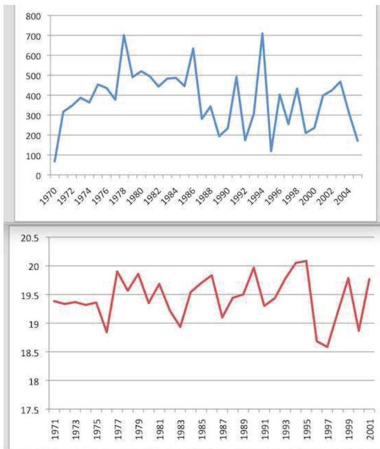
Γράφημα 2. Διαγράμματα βροχοπτώσεων (μπλε γραμμή) και μέσης θερμοκρασίας αέρα (κόκκινη γραμμή) από το 1970 έως το 2001 (Polymeni & Pafilis 2009).
