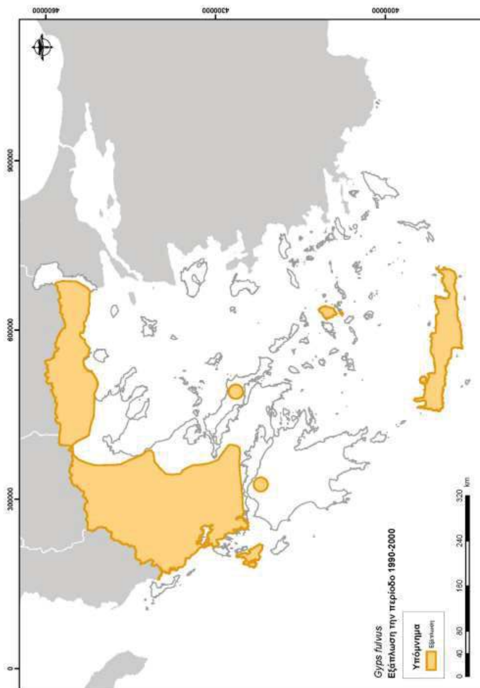
Χάρτης 3.2-3. Ζώνη εξάπλωσης του Όρνιου ( Gyps fulvus ) στην Ελλάδα την περίοδο 1990-2000 (κατά Bourdakis et al. 2006)
