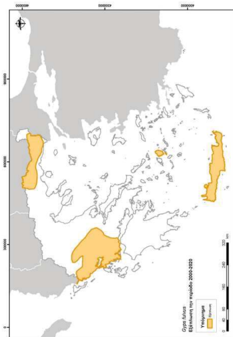
Χάρτης 3.2.2. Ζώνη εξάπλωσης του Όρνιου ( Gyps fulvus ) στην Ελλάδα την περίοδο 2000-2019 (κατά Λεγάκι & Μαραγκού 2009)
