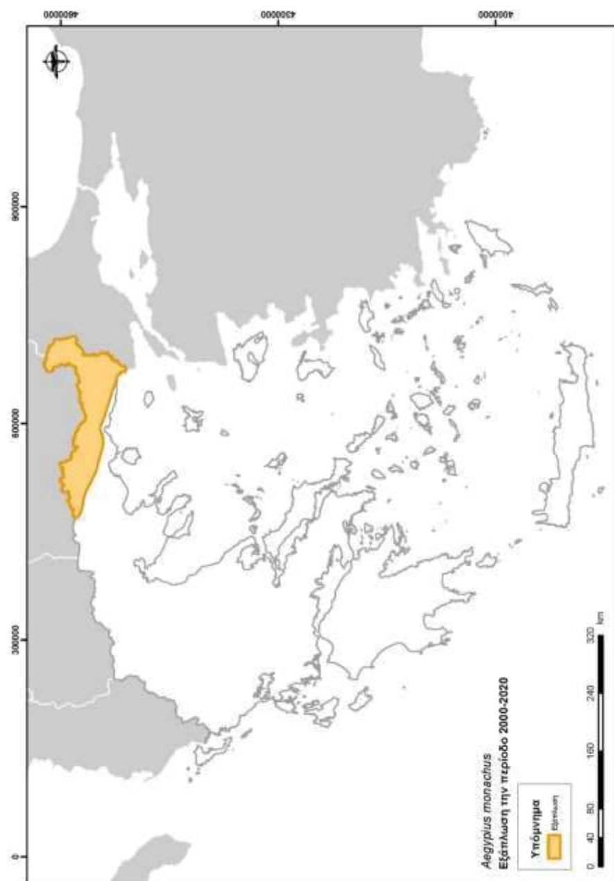
Χάρτης 3.3-2. Ζώνη εξάπλωσης του Μαυρόγυπα ( Aegypius monachus ) στην Ελλάδα την περίοδο 2000-2019 (κατά Bourdakis et al. 2006, Λεγάκις & Μαραγκού 2009).
