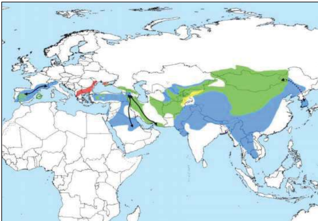
Χάρτης 3.3-1. Παγκόσμια εξάπλωση του Μαυρόγυπα ( Aegyrius monachus ) (κατά Botha et al. 2017).
