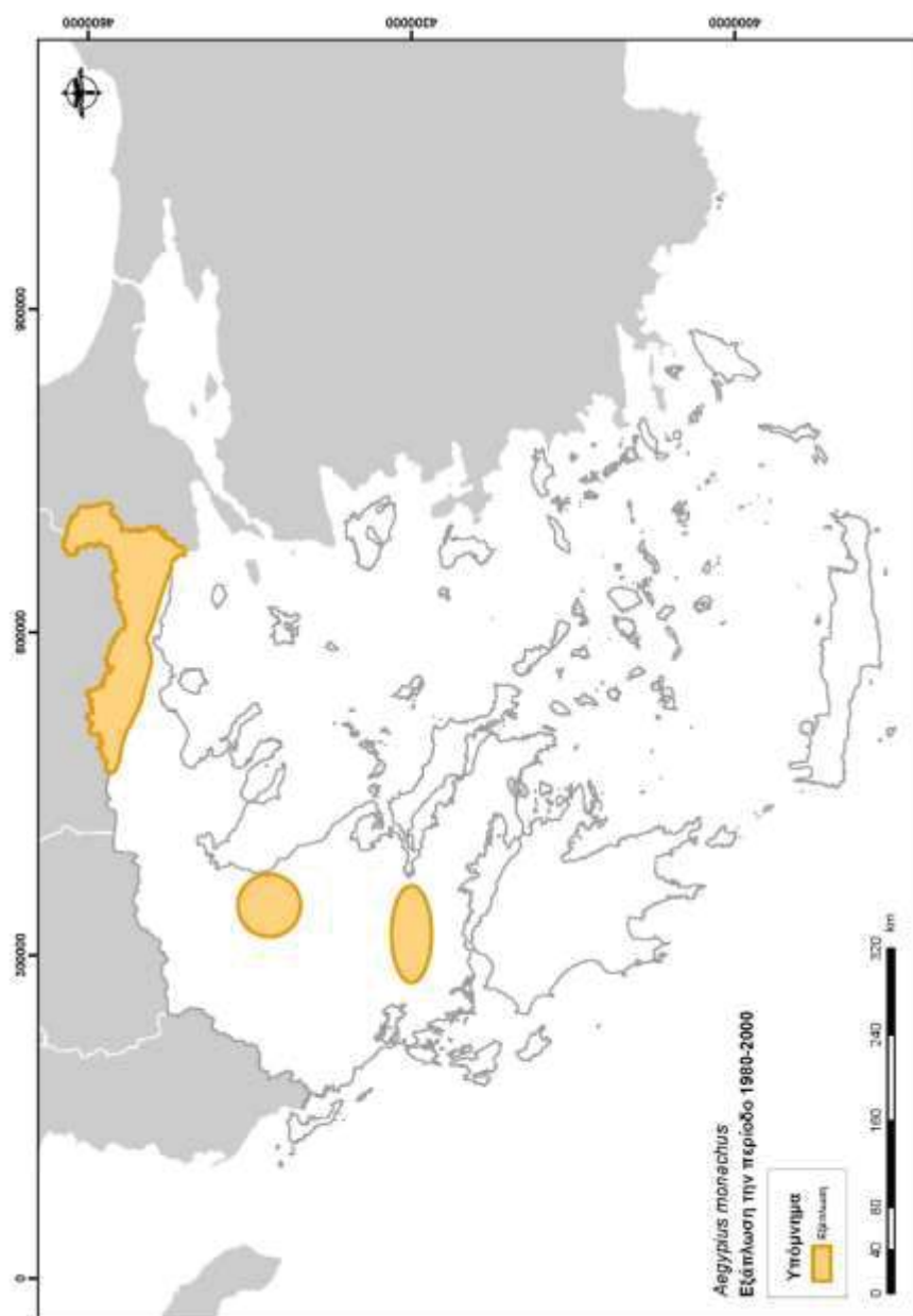
Χάρτης 3.3-3. Ζώνη εξάπλωσης του Μαυρόγυπα ( Aegypius monachus ) στην Ελλάδα την περίοδο 1980-2000 (Handrinos 1985, Bourdakis et al. 2006).
