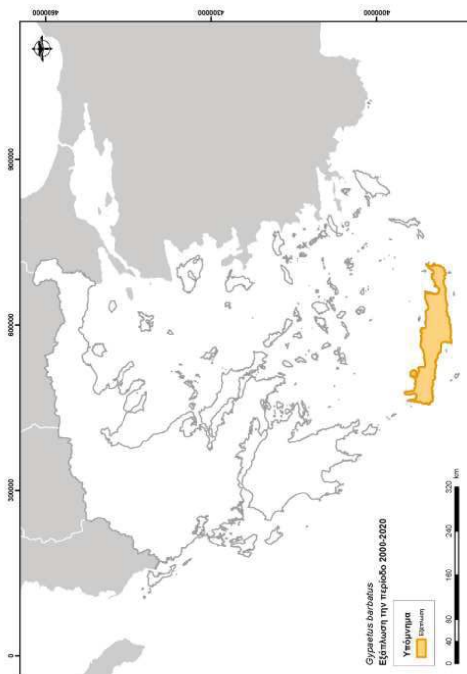
Χάρτης 3.1-2. Ζώνη εξάπλωσης του Γυπαετού ( Gypaetus barbatus ) στην Ελλάδα την περίοδο 2000-2020 (κατά Λεγάκις & Μαραγκού 2009).
