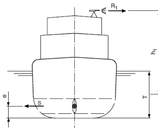
Σχήμα 7.2 Εγκάρσια αντίδραση της δέσμης νερού των εκτοξευτήρων πυρόσβεσης (firemonitors)
