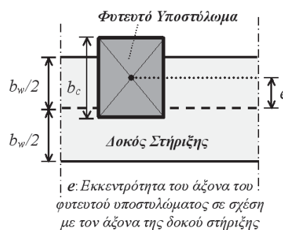
Φυτευτό υποστυλώμα έκκεντρα στηριζόμενο σε δοκό (ΚΑ 3 )
