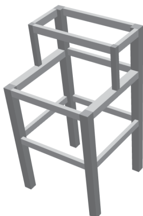
Φυτευτό υποστυλώμα έκκεντρα στηριζόμενο σε δοκό (ΚΑ 3 )
