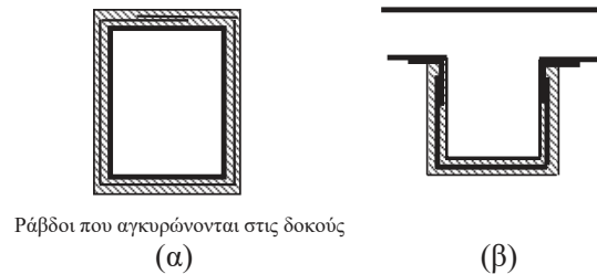
Σχ.Σ8.3: Ενδεικτικοί τρόποι ενίσχυσης σε διάτμηση έναντι ανεπάρκειας σε λοξή θλίψη: (α), Κλειστές ενισχύσεις, (β) Ανοικτές ενισχύσεις με ισχυρή σύνδεση στα άκρα
