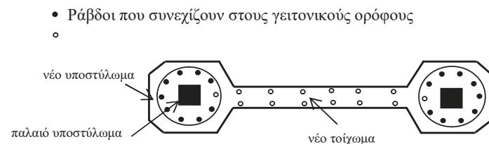
Σχ. Σ8.6: Ενδεικτική εμφάντωση με πάχος ίσο ή μικρότερο του πλάτους της δοκού
