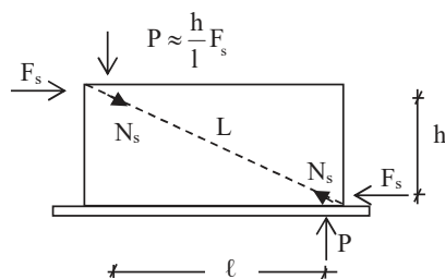
Σχ. Σ8.7: Τέμνουσα φατνώματος
