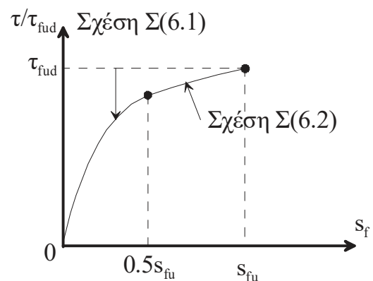
Σχ. Σ6.3: Διάγραμμα διατμητικών τάσεων-σχετικών ολισθήσεων κατά μήκος τραχειάς διεπιφάνειας σκυροδέματος (σχηματικό).
