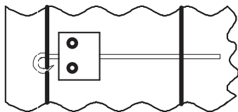
Σχ. Σ8.10: Ενδεικτική απεικόνιση αγκύρωσης οριζόντιων οπλισμών.
