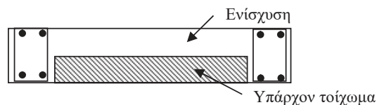
Σχ. Σ8.4: Ενδεικτική διάταξη μονόπλευρης ενίσχυσης τοιχώματος
