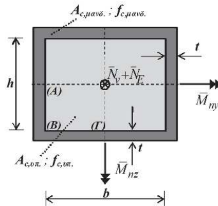
Σχ. Σ8.Α: Μανδύας υποστυλώματος.
