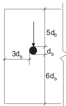
Σχ. Σ6.6: Ορισμός επικαλύψεων βλήτρου
