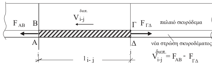
Σχ. Σ8.2: Διατμητική δύναμη στη διεπιφάνεια
