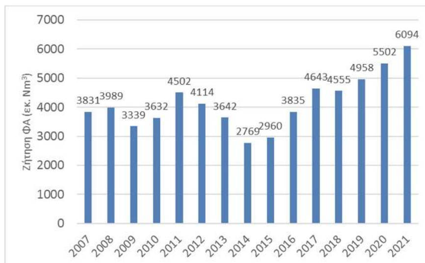
Γράφημα 8: Ζήτηση ανά κατηγορία καταναλωτών για τα έτη 2007 - 2021, φυσικές εγχύσεις στο σύστημα (πηγή: ΔΕΣΦΑ - Μελέτη Ανάπτυξης ΕΣΦΑ 2021-2030)
