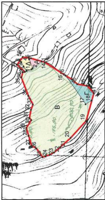
Φύλλο χάρτη Γ.Υ.Σ. 6466/7 Κλ.Χάρτη 1:5000
